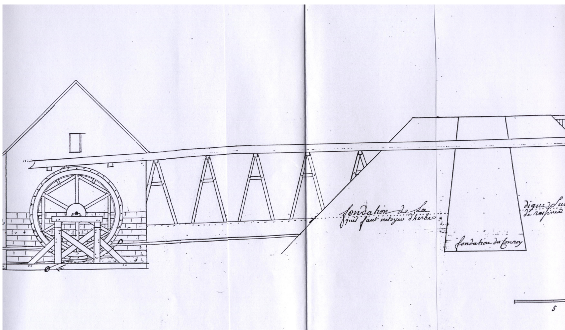
Moulin de Saint-Amand-des-Hautes-Terres en 1751. Collection particulière.
